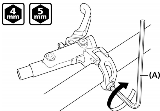
(A) Clé à six pans de 4 mm/ Clé à six pans de 5 mm
