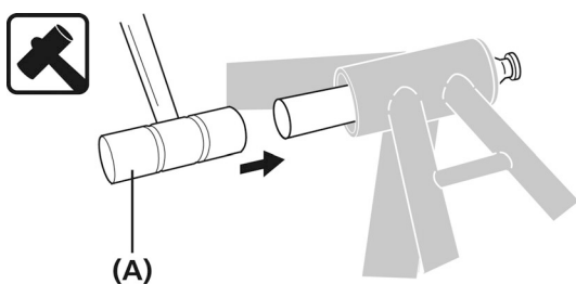
(A) Maillet en plastique
