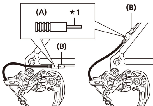
(A) Bouchon extérieur étanche avec languette
