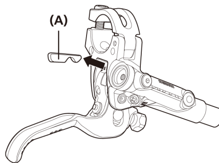
(A) Butée de manette
