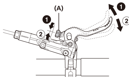
(A) Boulon de réglage d'extension
