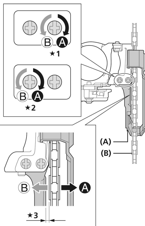
★1 Dérailleur Top swing
