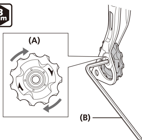
(A) Galet de tension
